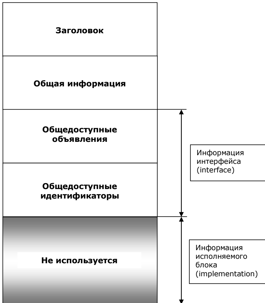
Рисунок А1. Форма файла PPU.
