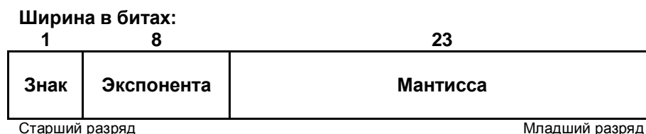
Рис. 8.1. Формат single .
