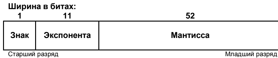
Рис. 8.2. Формат double.
